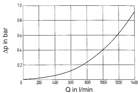
RFLD 951 ... 1301
