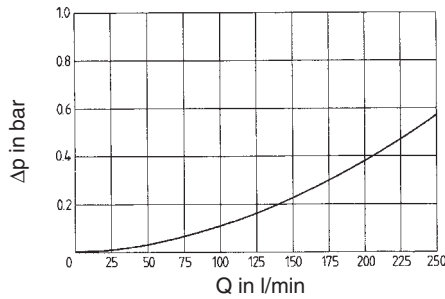
RFLD 331 ... 501
