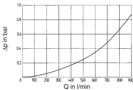
RFLD 951 ... 1301
